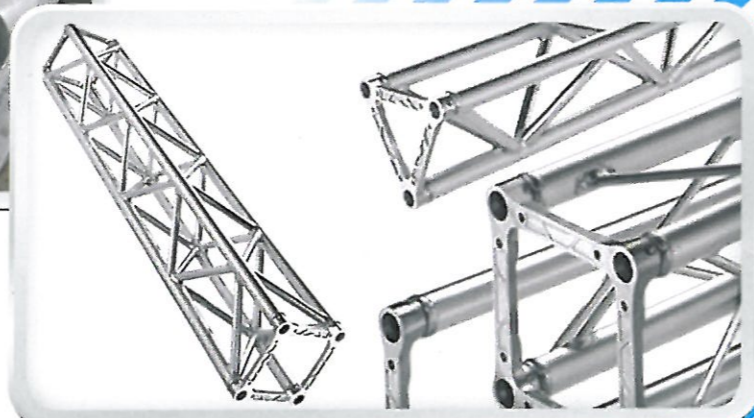
SALDATE DI STRUTTURE IN ALLUMINIO
